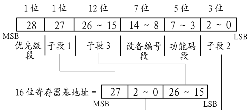
图 10-1： TTCANopen ID 划分方案
